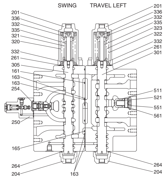
SECTION D-D
